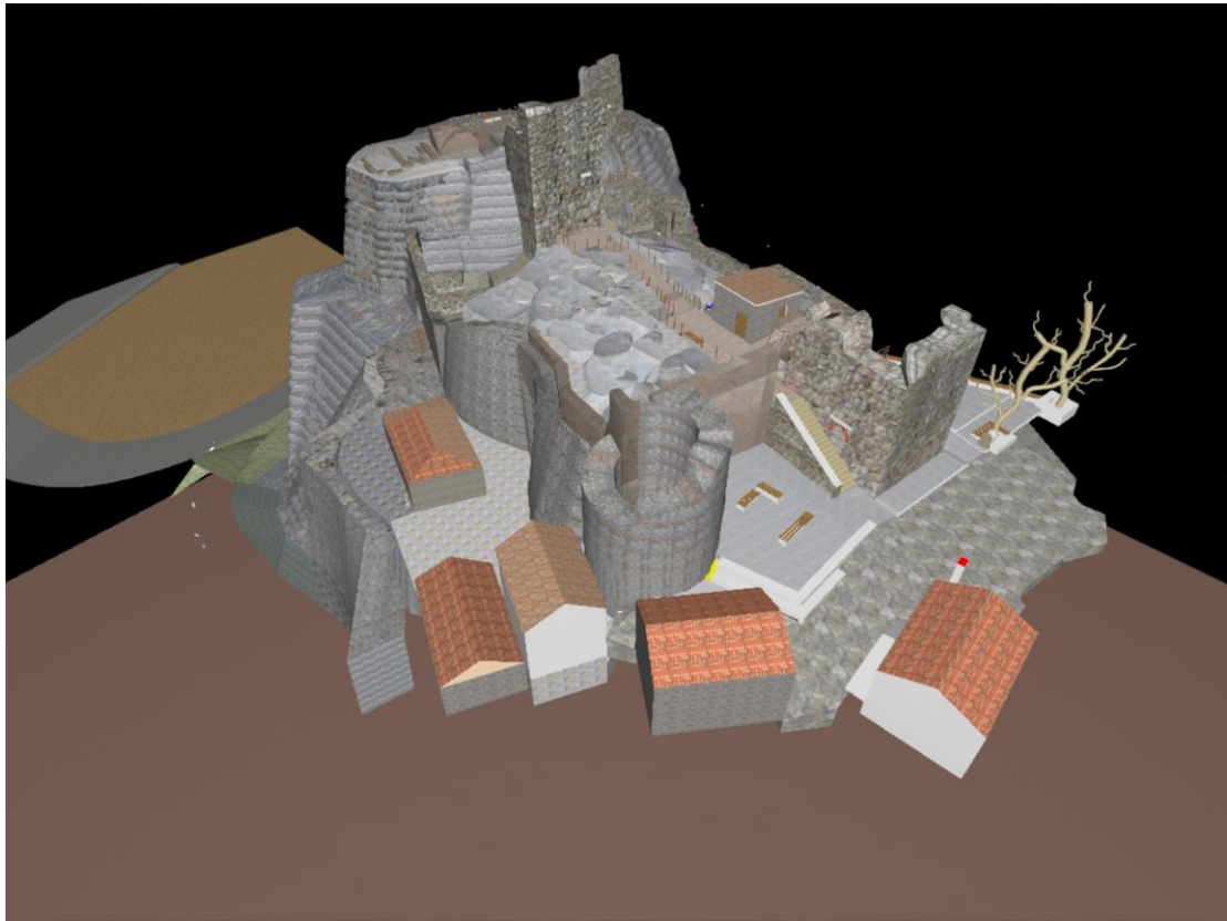
Εικ. 1 Κάστρο Σαμοθράκης. Τρισδιάστατη απεικόνιση
